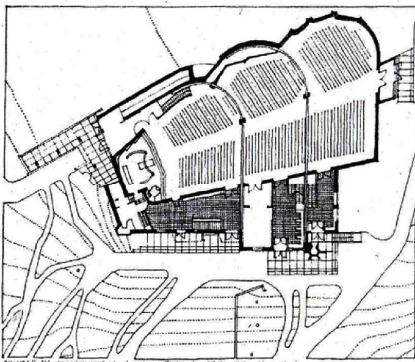
CHURCH IN VUOKSENENKA, Imatra, Finland. 1958-60. Alvar Aalto
