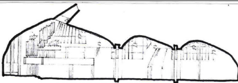
CHURCH IN VUOKSENENKA : Imatra, Finland. 1958 Alvar Aalto
