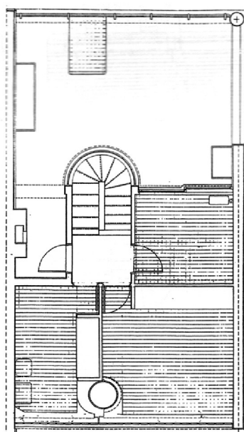
► PLAN R+1
