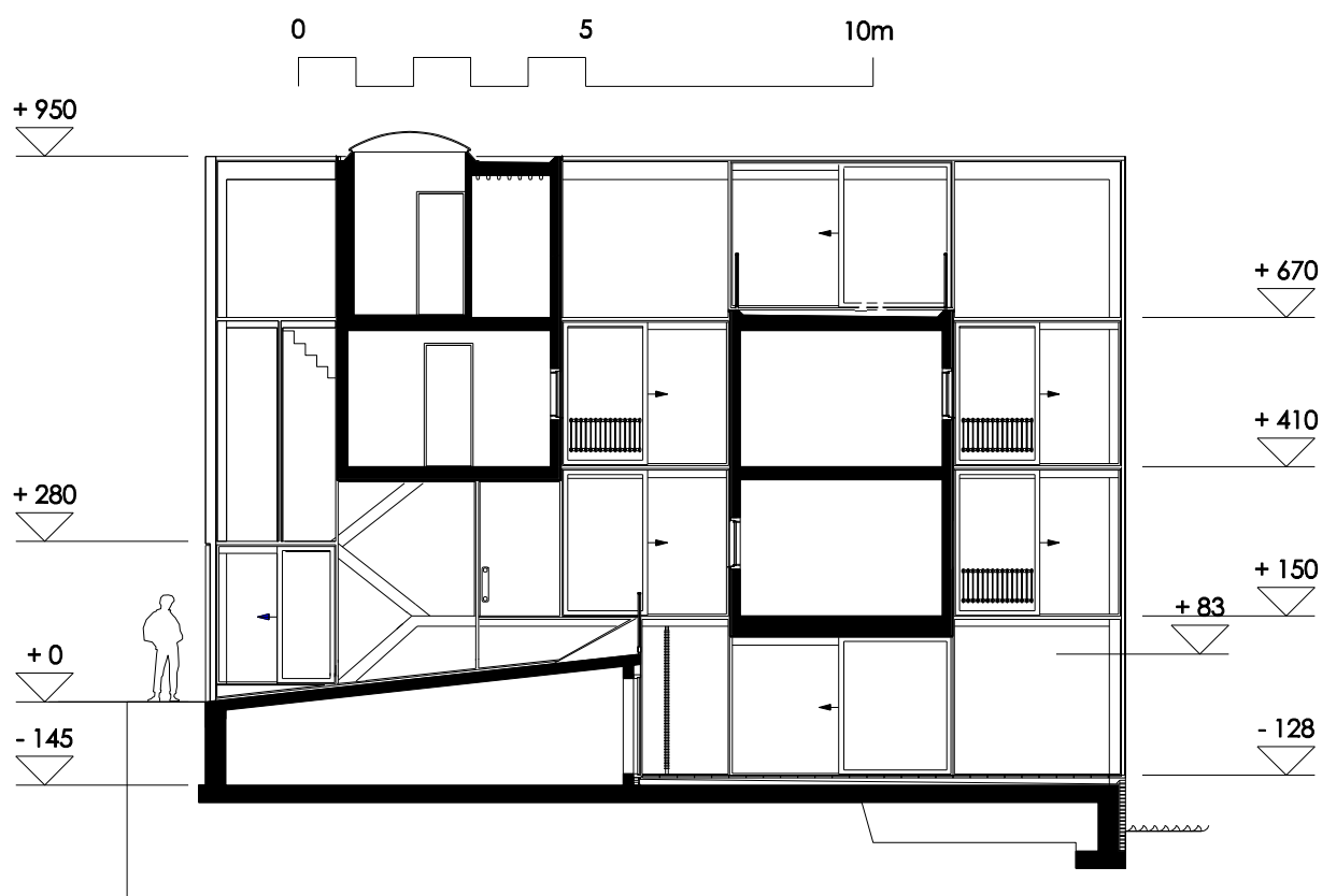
► COUPE LONGITUDINALE
