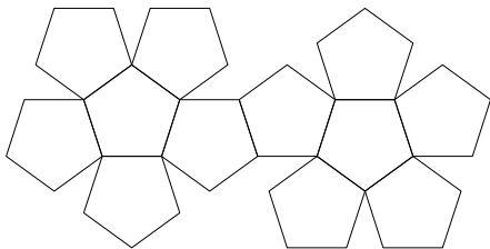
Dodécaèdre
