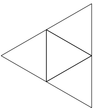
Tétraèdre
