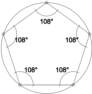
Pentagone régulier
