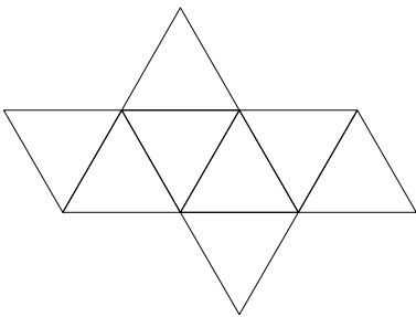
Octaèdre
