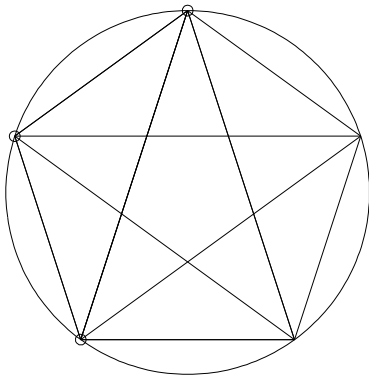
Un des triangles d'or "obtus" du pentagone
