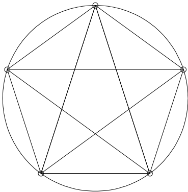
Pentagramme (ou "pentagone étoilé") inscrit dans le pentagone
